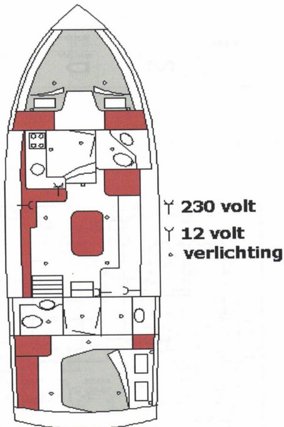
Afbeelding B11-1: 24 - 230 Volt met aansluitpunten
